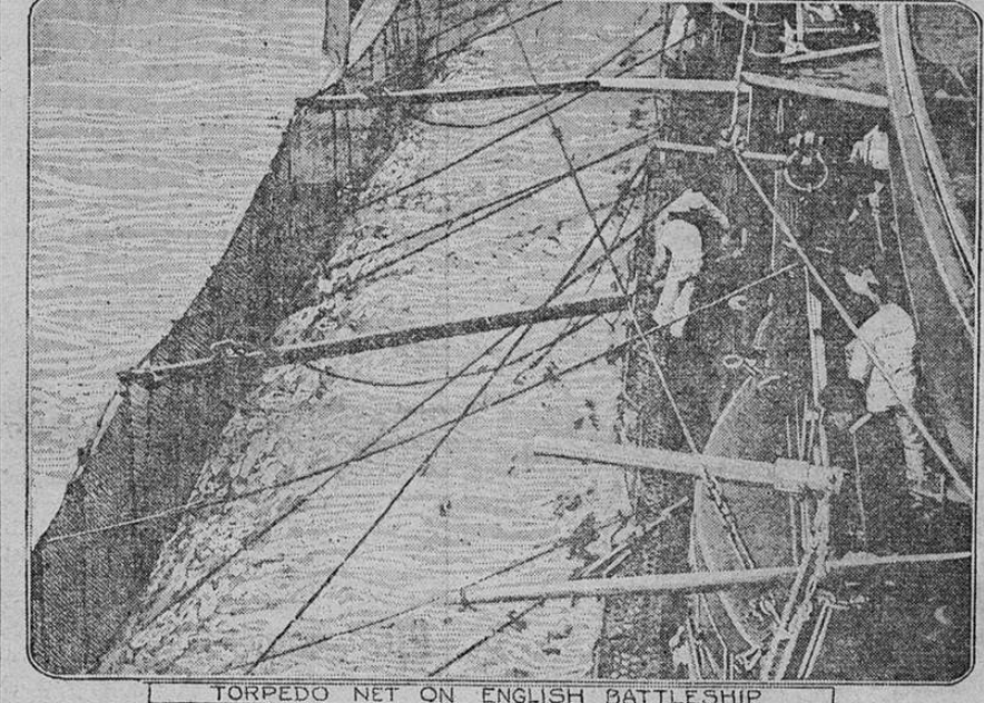
TORPEDO NET ON ENGLISH BATTLESHIP El superdreadnought británico IRON DUKE está protegido por una enorme red extendida al rededor del buque sobre botafonías (palos largos que se sacan hacia la parte exterior de una embarcación, cuando conviene, y que son destinados a varios usos) cuya red avanza suficientemente en el agua para detener los torpedos. La red es usada como medio de acción en la noche y es preferentemente aplicada en aguas hostiles y cuando se considera que hay peligro de minas flotantes en la línea adoptada para el tránsito del navio.
